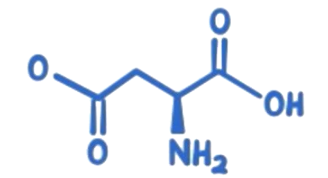
АСПАРАГІНОВА КИСЛОТА
