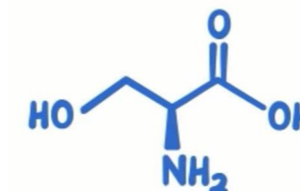
СЕРИН
