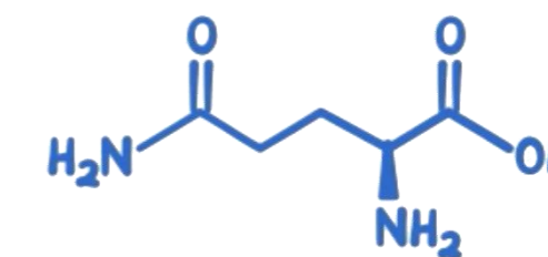
ГЛЮТАМІН
