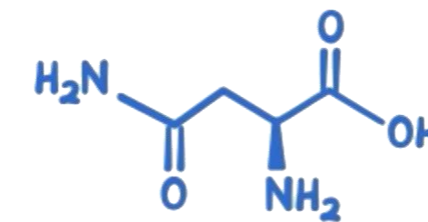
АСПАРАГІН
