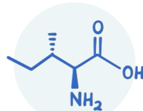
ІЗОЛЕЙЦИН
