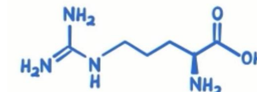
АРГІНІН
