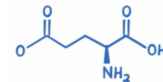
ГЛЮТАМІНОВА КИСЛОТА
