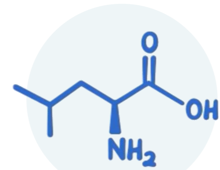
ЛЕЙЦИН
