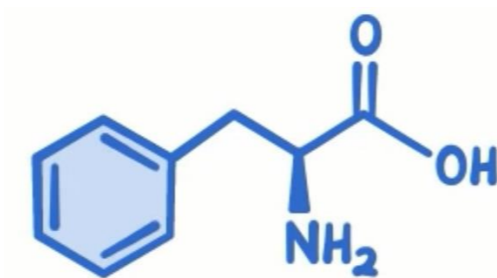
ФЕНІЛАЛАНІН
