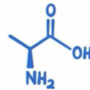
АЛАНІН
