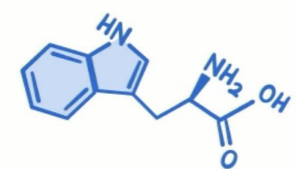
ТРИПТОФАН
