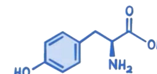
ТИРОЗИН
