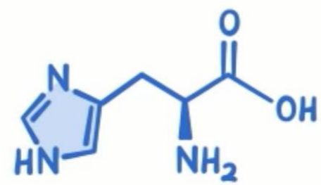
ГІСТИДИН
