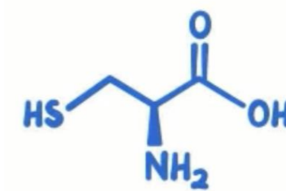
ЦИСТЕЇН
