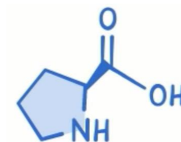
ПРОЛІН
